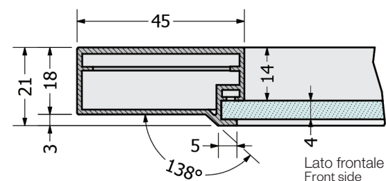
SEZIONE TECNICA ANTA "PRISMA" "PRISMA" DOOR TECHNICAL SECTION
