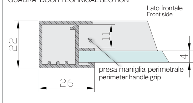
SEZIONE TECNICA ANTA "QUADRA" "QUADRA" DOOR TECHNICAL SECTION
